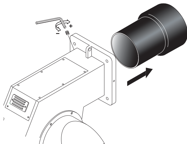
ДЕМОНТАЖ СТАКАНА
